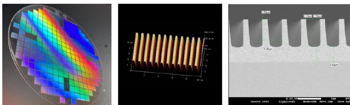
図 4-60 200mm ガラスウェハー上にインプリント形成された高屈折率ポリマーを使ったハイアスペクト比の矩形パターン。
