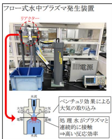
図2-4 プラズマ発生装置
